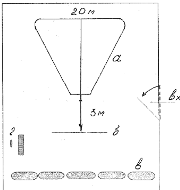
Рис. 1. Выводная площадка
